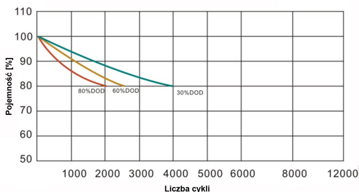
Żywotność w zależności od głę. rozładowań przy 25°C i 0.2C
